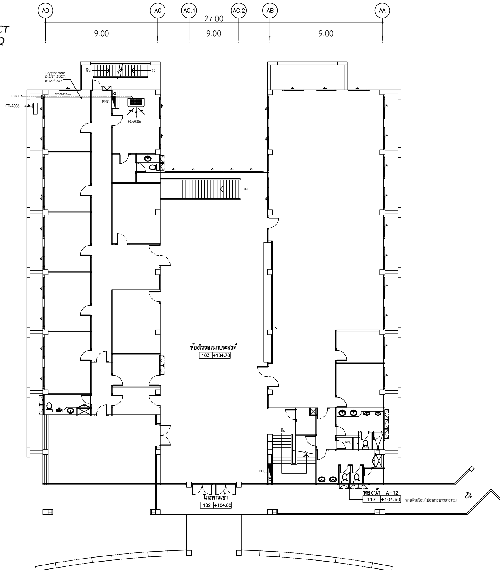
แบบระบบเครื่องปรับอากาศ 1st FLOOR PLAN
