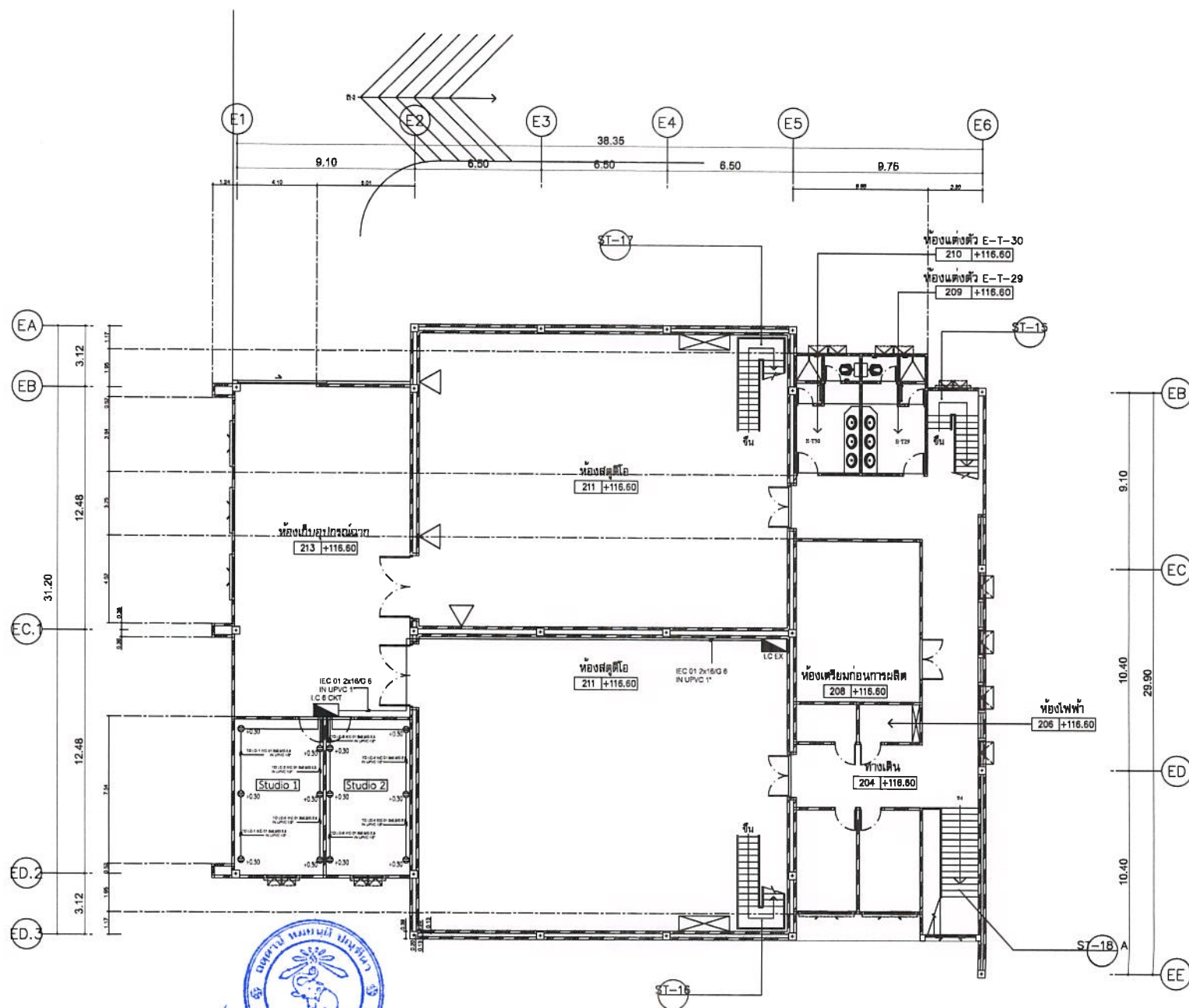
แบบแสดงงานเดินไฟฟ้า 1
